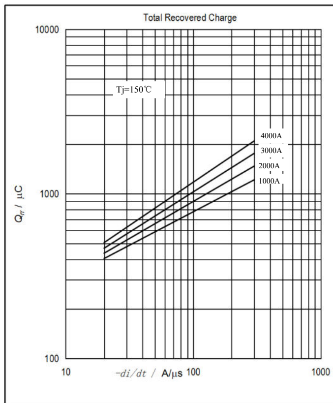
图5. 恢复电荷与电流变化率的关系曲线
