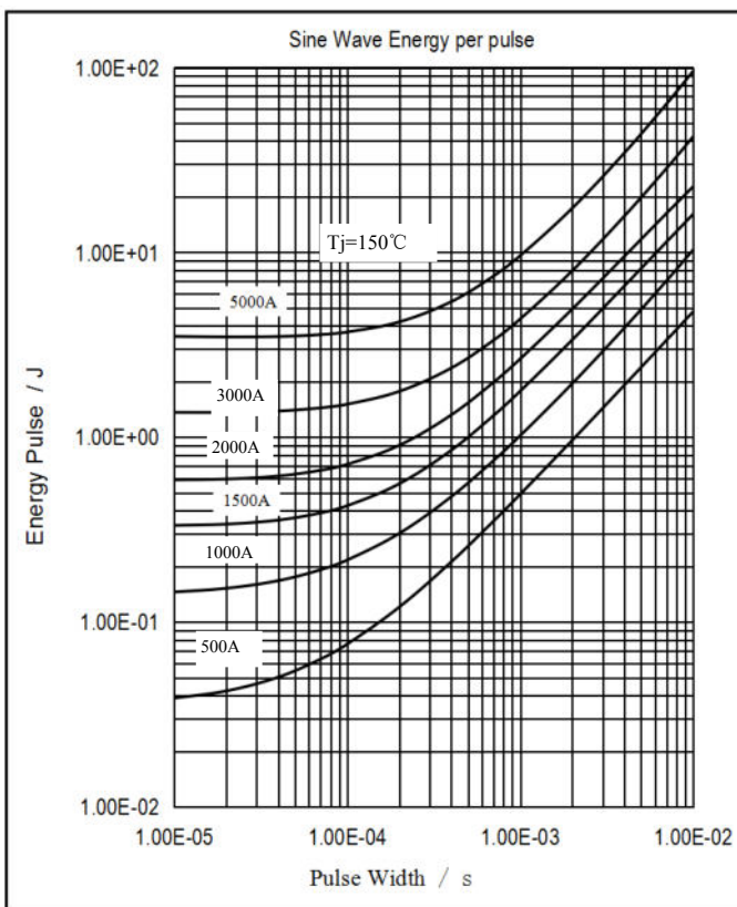
图6. 正弦波能量与脉宽的关系曲线
